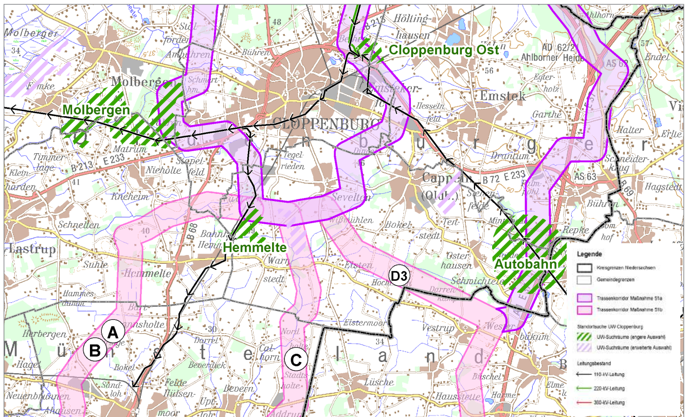
Abb. 38: Übersicht über mögliche Trassenführungen und Suchräume für Umspannwerke (Stand: 21.09.2016)
